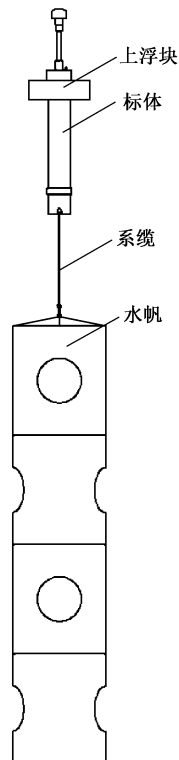
图 B.1 表层漂流浮标的结构示意图
